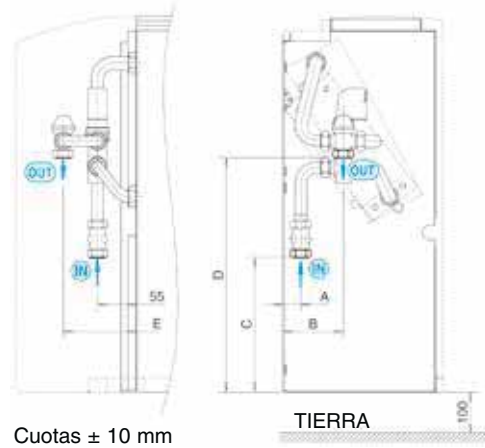
Cuotas ± 10 mm
