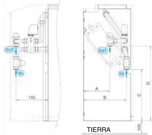
Cuotas ± 10 mm
