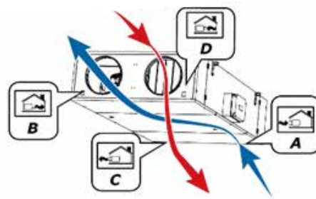
Configuração de fluxos invertidos de teto
