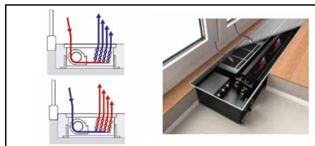
Convecção forçada com 4 tubos para frio e calor
