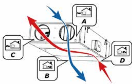
Configuração padrão de teto
