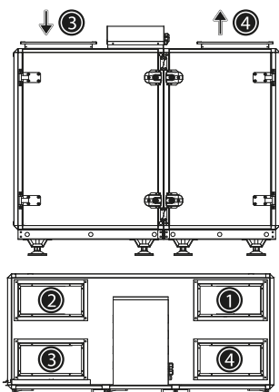
Configuración izquierda
