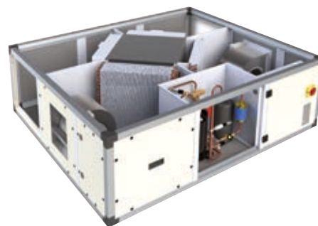
Recuperador termodinámico TECNA SIC CFR-HP
